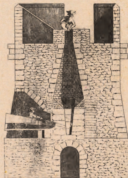
▲ Przekrój wielkiego pieca z końca XVIII w., Aleksander Bocheński, Wędrówki po dziejach przemysłu polskiego , Warszawa 1966
